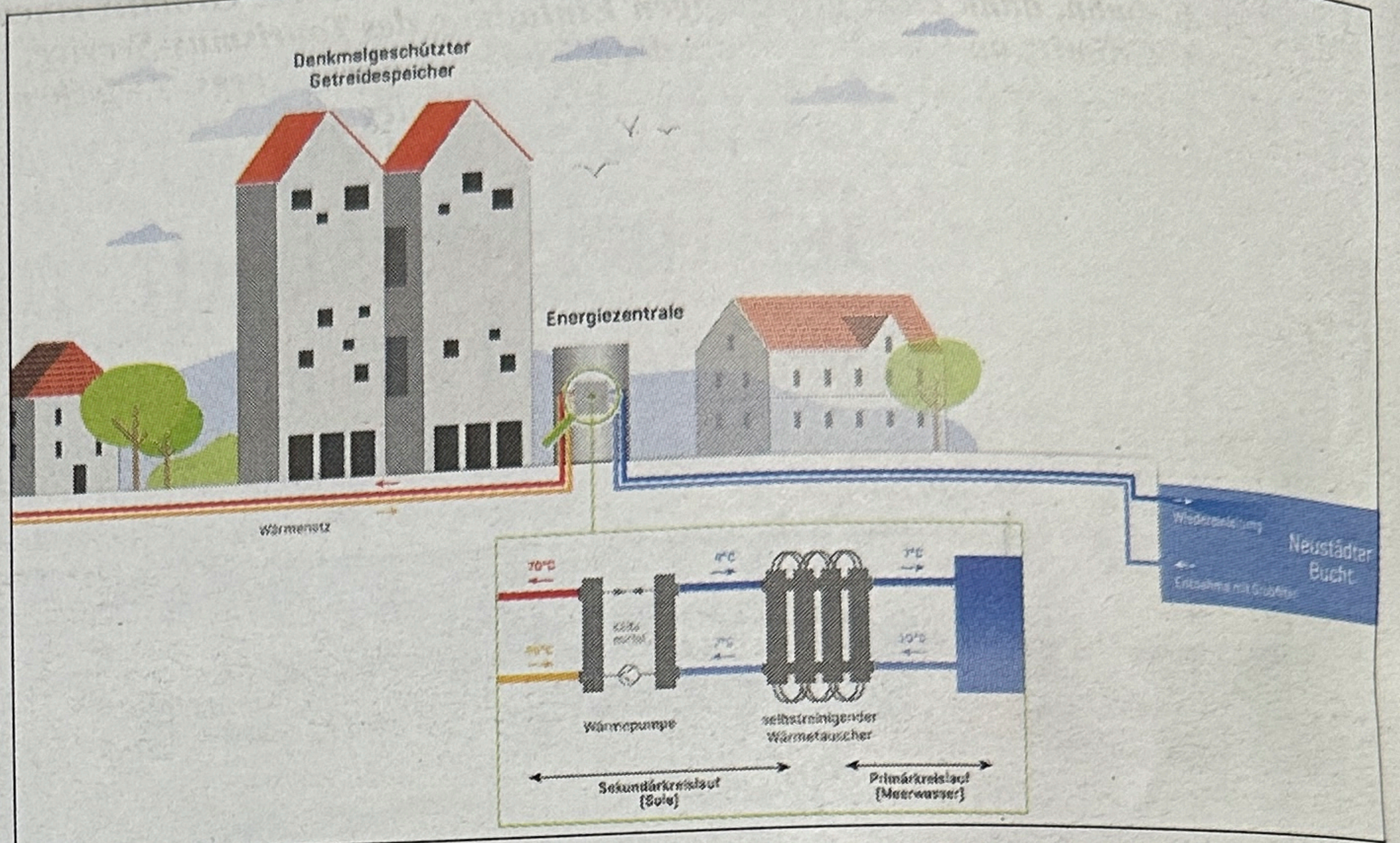
Funktionsweise der Meerwasser-Wärmepumpe. (Foto: Hamburg Institut)
